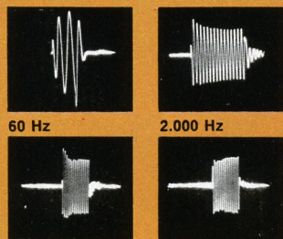
8.000 Hz 16.000 Hz Livello a 1 metro 2,83 Volt, rumore rosa 88,2 dB
