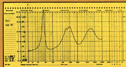
Modulo dell'impedenza
