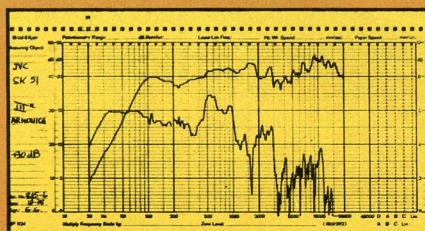
Risposta in frequenza sull'asse e distorsione di terza armonica
