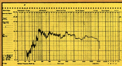
Risposta in frequenza in ambiente
